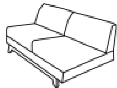
Love sin brazos Frente: 154 cm Fondo: 90 cm Alto: 75 cm
